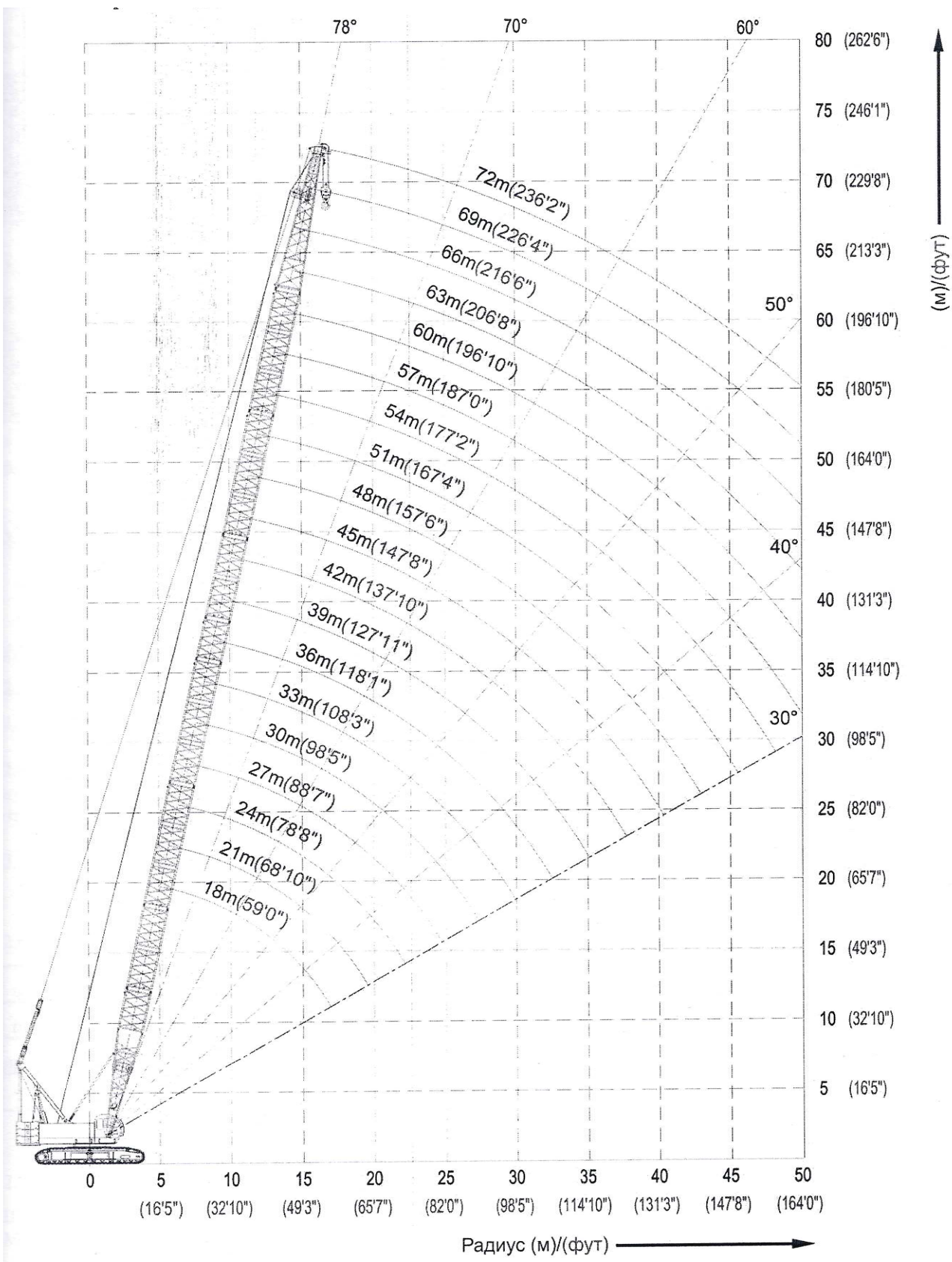
Рис. 4. Высотные характеристики крана без гуська
